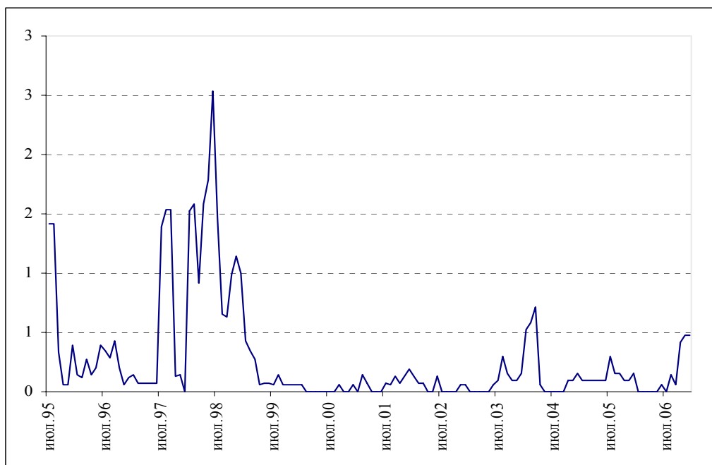
Рисунок 3. Динамика индекса I^3 в июле 1995 – декабре 2006 гг.
