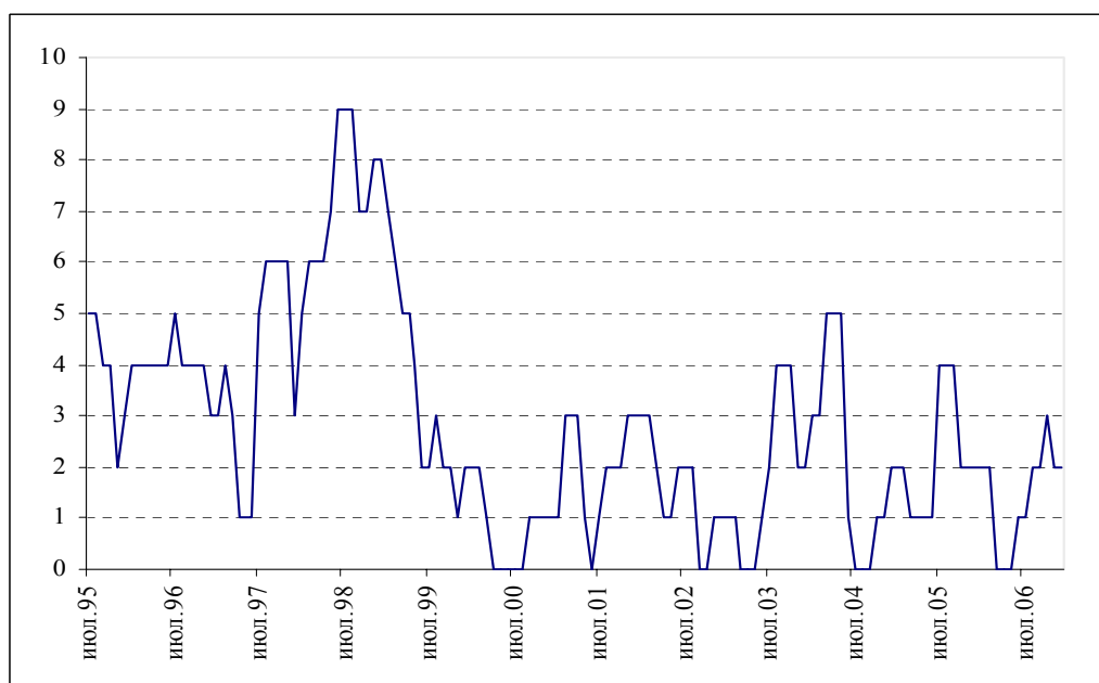
Рисунок 2 Динамика индекса I^2 в июле 1995 – декабре 2006 гг.
