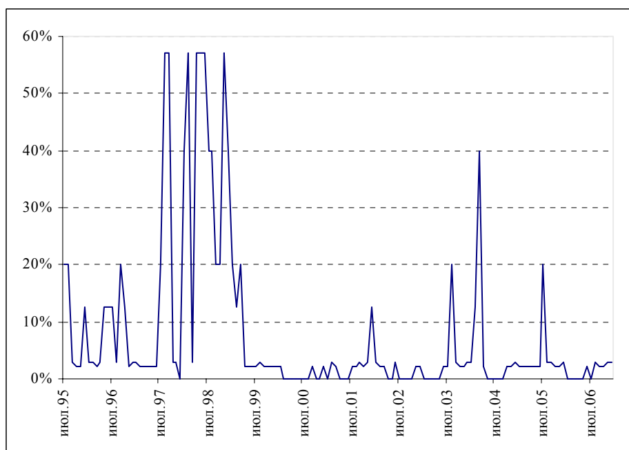
Рисунок 4. Оценка вероятности наступления финансовой нестабильности в июле 1995 – декабре 1996 гг. с помощью индекса I^1 .
