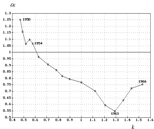
Рис.3.7. Пример зависимости (\varepsilon_K, k) .
