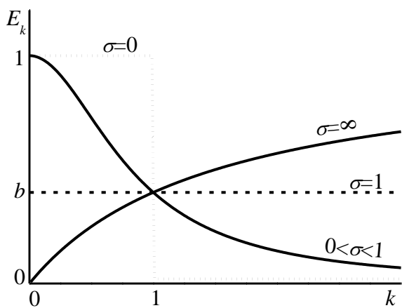
Рис.2.5. Зависимости (E_k,k) для разных значений эластичности замещения \sigma .
