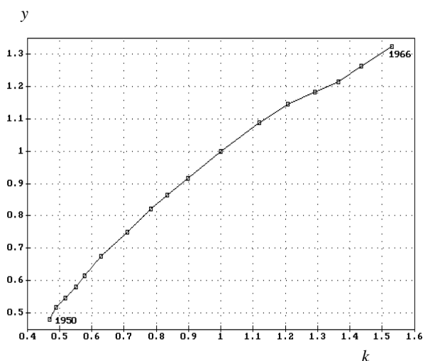
Рис.3.3. Пример зависимости (y,k) .
