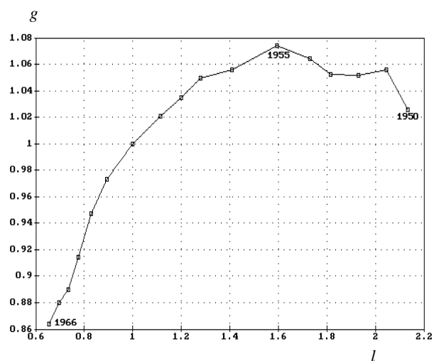
Рис.3.4. Пример зависимости (g,l) .
