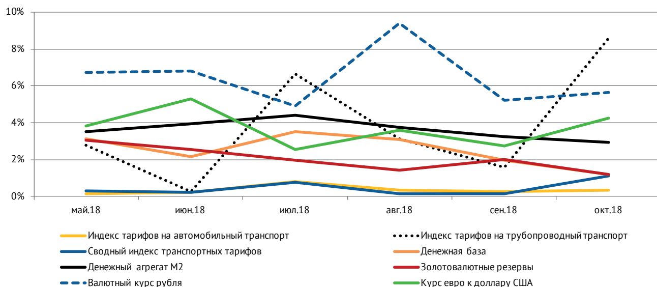
Рис. 1. Средняя абсолютная процентная ошибка прогнозов в мае-октябре 2018 г.
